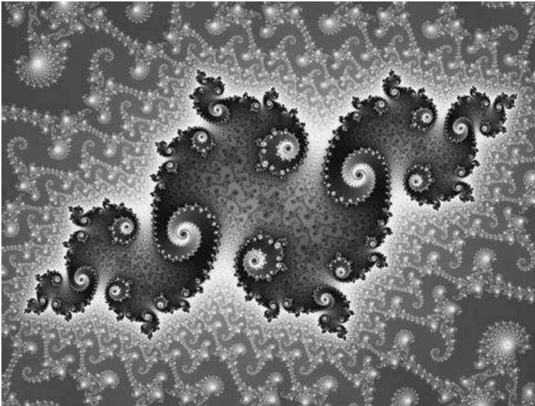
Вариант изображения множества Мандельброта — результата многократного повторения простой математической формулы. При приближении к какой-либо точке кажется, что изображение постоянно меняется непредсказуемым образом.
